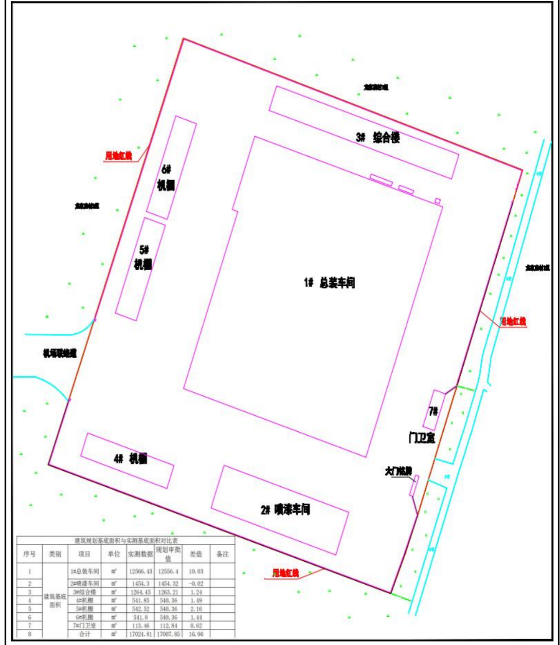
竣工实测项目平面图
